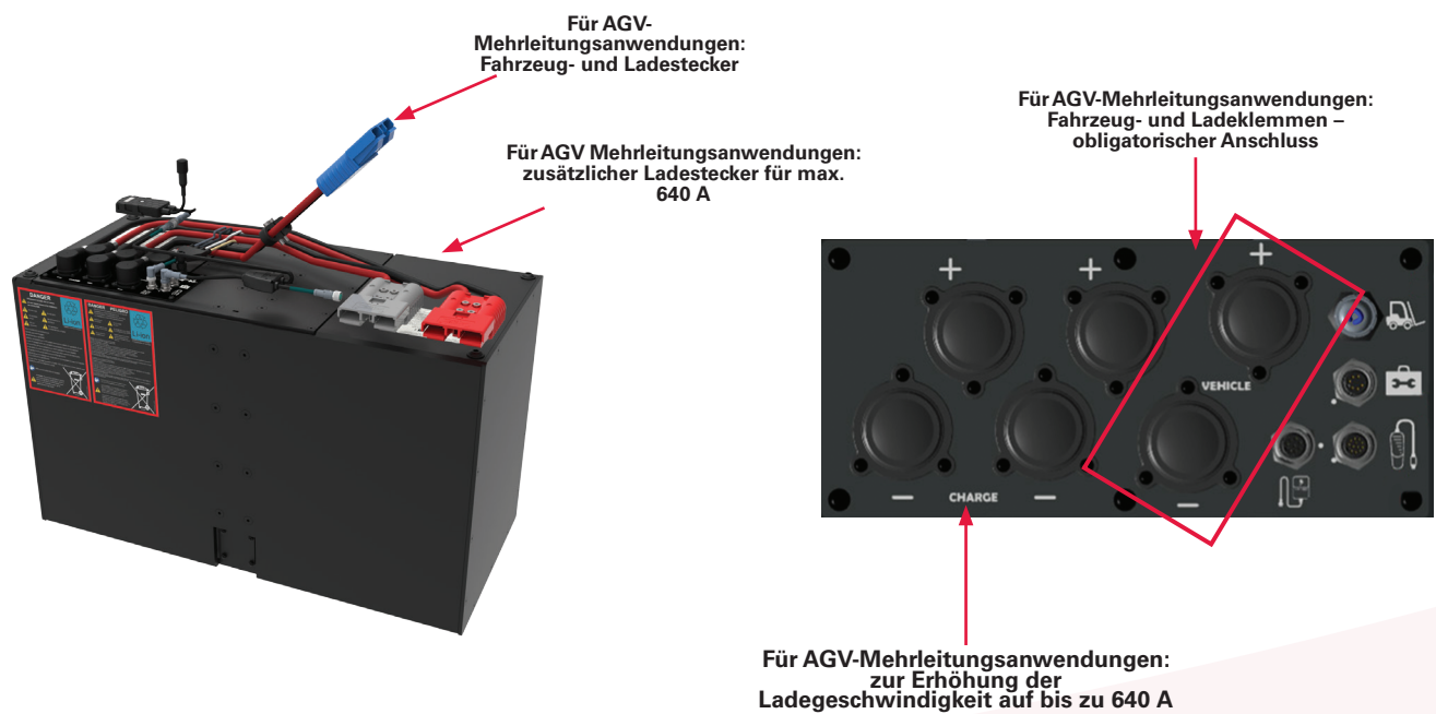
Abbildung 5: AGV-Mehrleitungsanwendung
