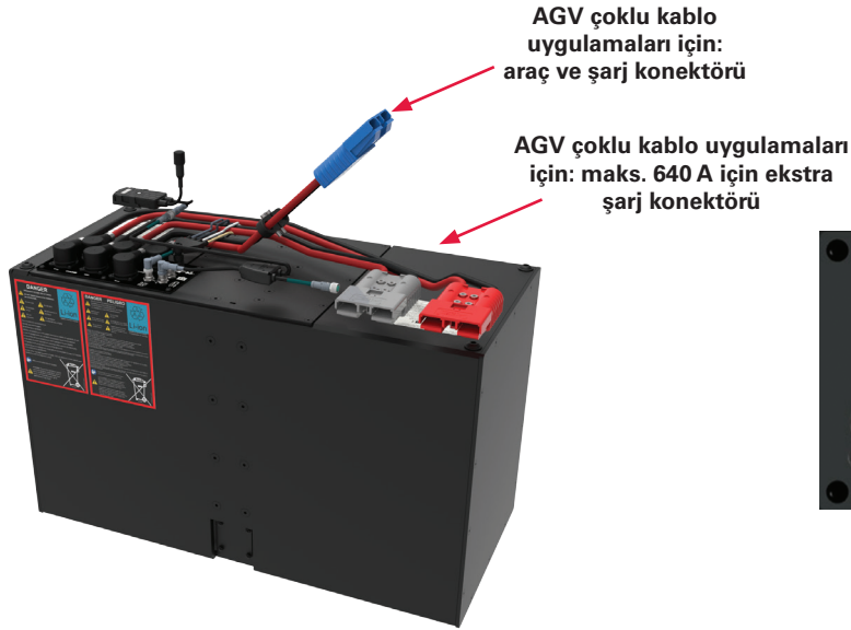
Şekil 5: AGV Çoklu Kablo Uygulaması
