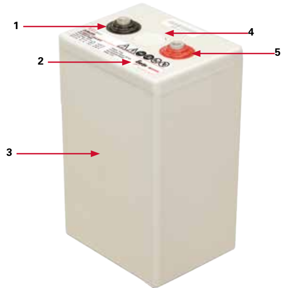
Delene på en 2V ZeMaRail™ enkeltcelle
