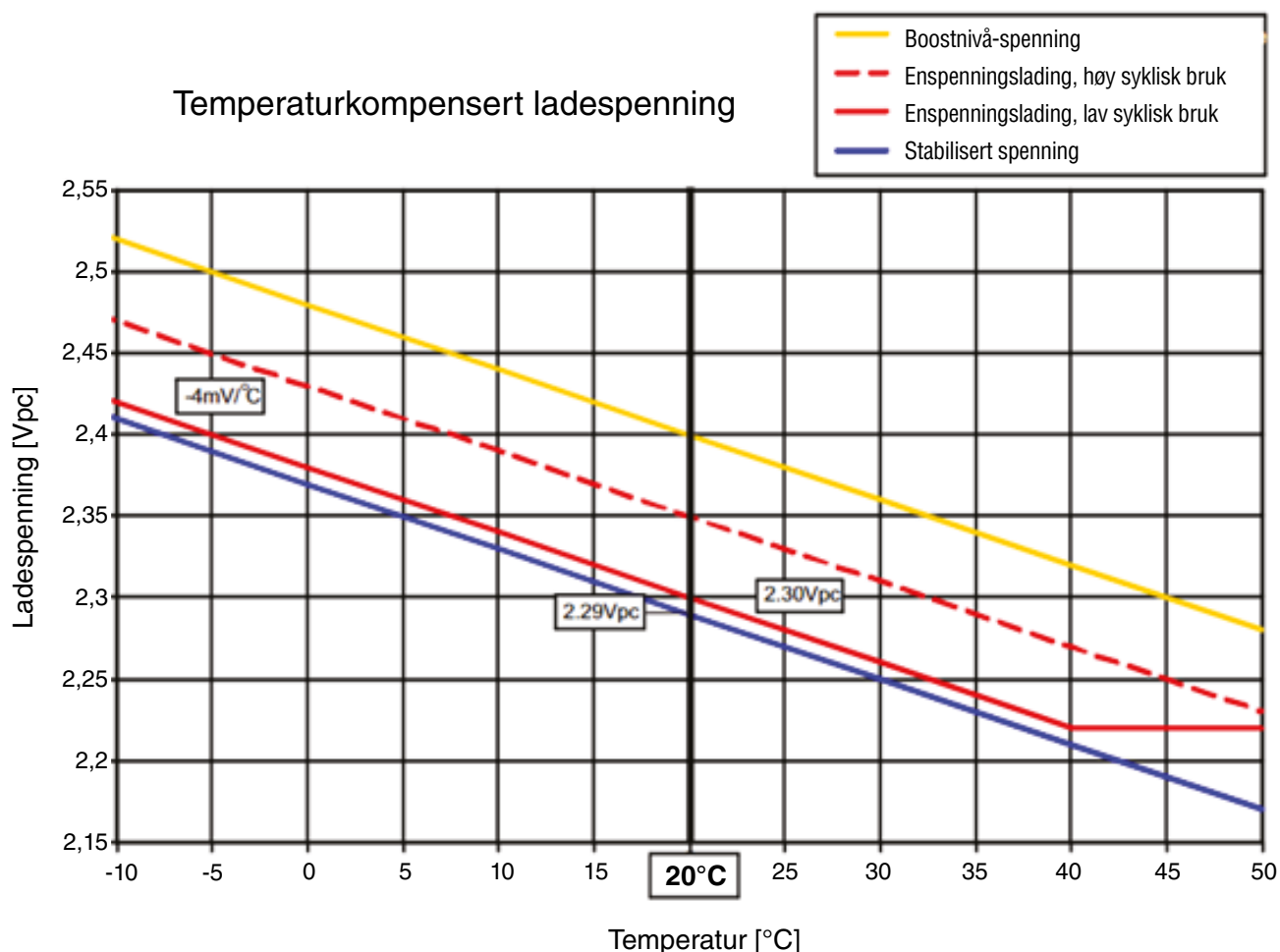
Figur 4: Temperaturkompensert ladespenning
