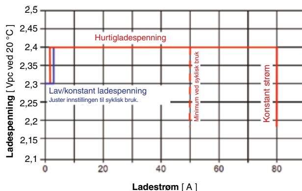
Figur 3: Lade karakteristikk IU0U-lading for ZeMa200P18*
