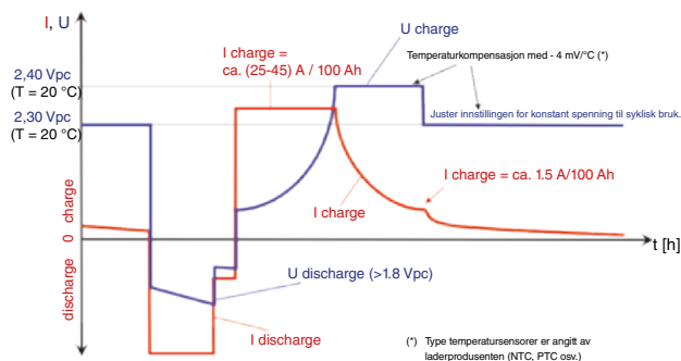
Figur 2: Driftsmodusene "charge-discharge-charge" med lade karakteristikk "IU0U"
