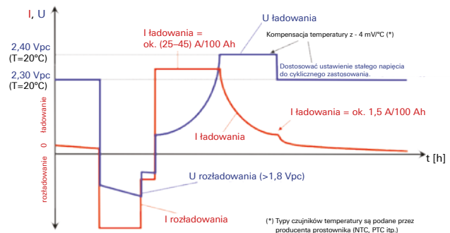
Rys. 2: Tryby działania ładowanie-wyładowanie-ładowanie z charakterystyką ładowania IUOU
