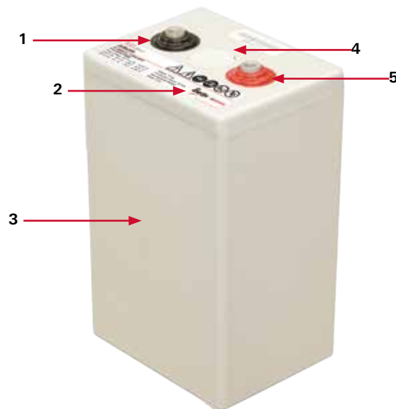
Części pojedynczego ogniwa ZeMaRail™ 2 V
