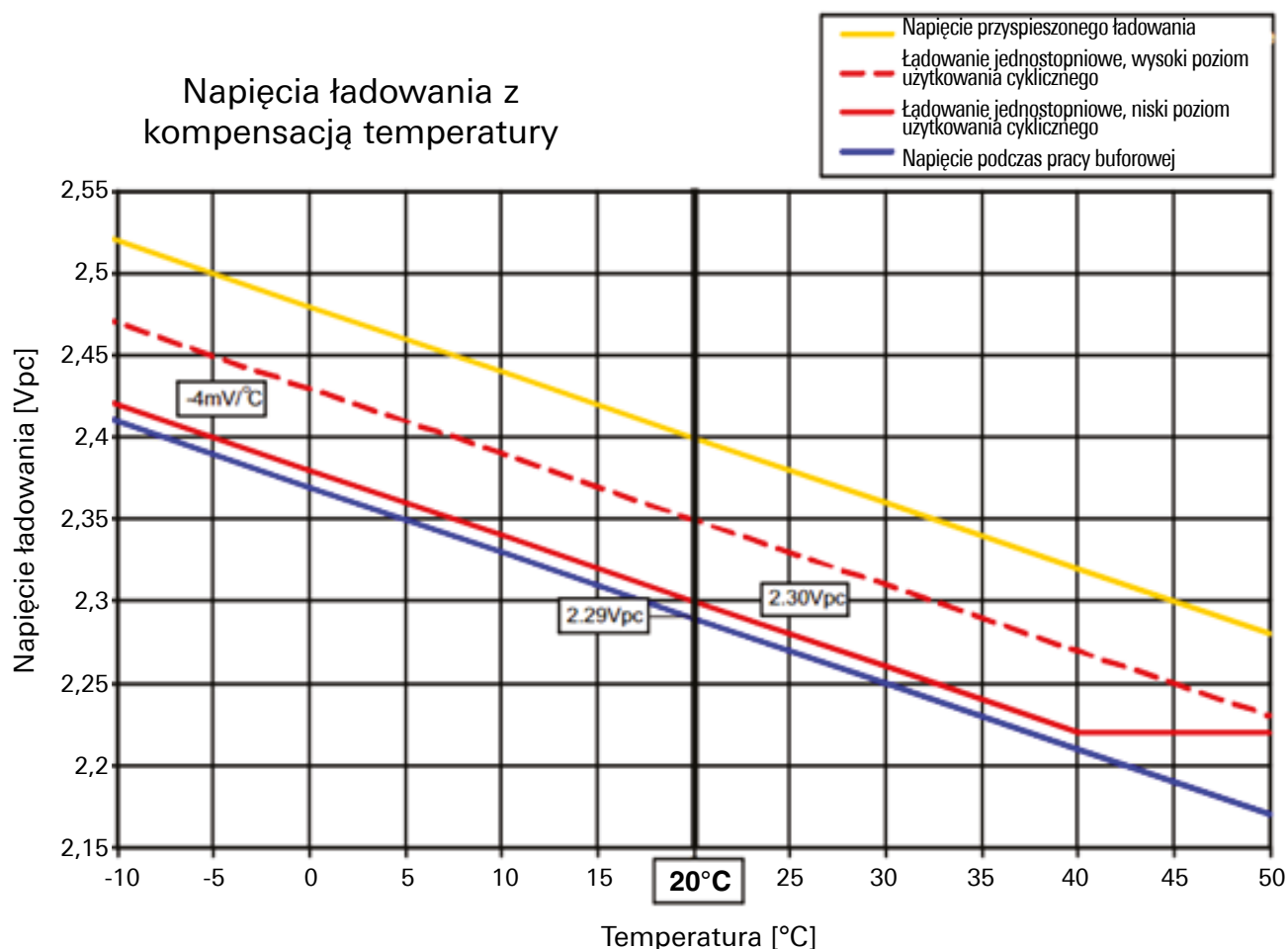
Rys. 4: Napięcia ładowania z kompensacją temperatury
