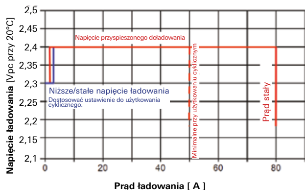
Rys. 3: Charakterystyka ładowania IU0U dla ZeMa200P18*
